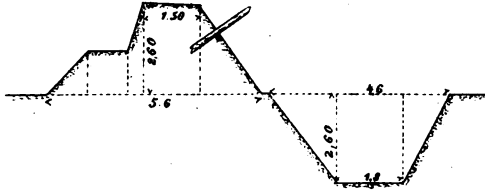
Profiel van de Contravallatie Linie 1 200
